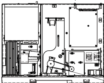
Top view without cover/ Vue de dessus sans capot
