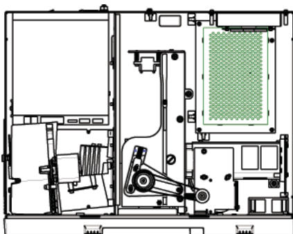
Top view without cover/ Vue de dessus sans capot
